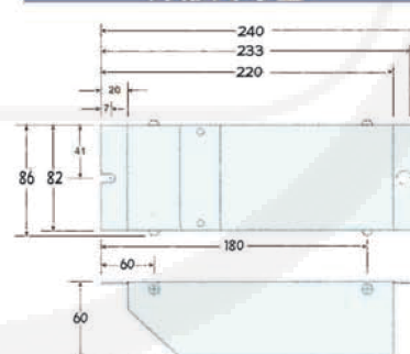
外部尺寸圖
