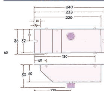
外部尺寸圖
