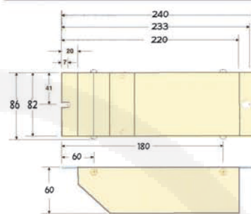
外部尺寸圖
