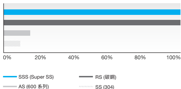
最大可容許張力(MAL)額定值
