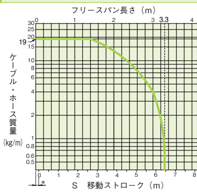
HSB△△ (プラスチック) △△=CあるいはD寸法
