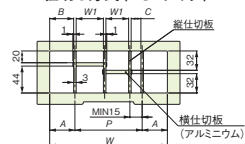
④一部分を上下2段あるいは3段に仕切る方式 (DSBタイプ)
