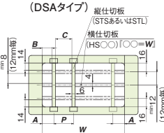
② 全体を上下多段に仕切る方式 (DSAタイプ)
