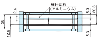
④ 上下3段に仕切る方式 (DSA・DSBタイプ共通)
