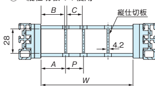
① 縦仕切板のみ使用
