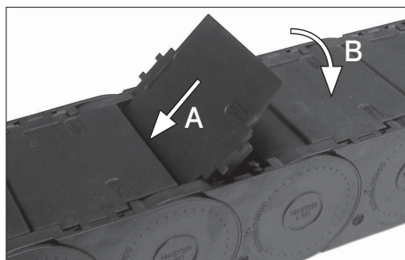
①カバーを矢印 A の方向に挿入し、矢印 B の方向に回転させます。
