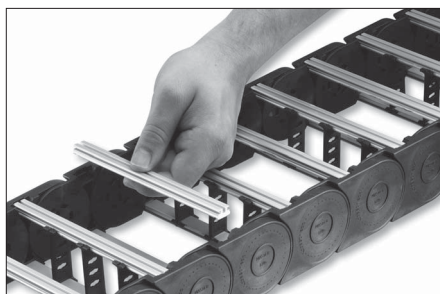
③ステイが外れます。
