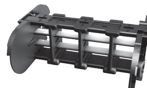
■仕切板取り付け状態例 (DSAタイプ)
