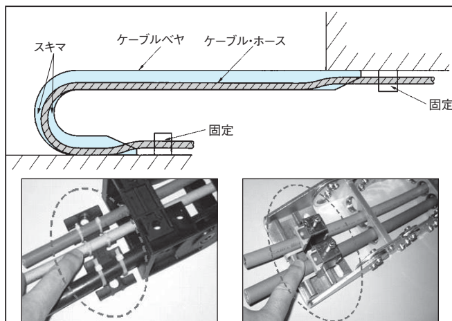
図5 ケーブル・ホースの固定方法例
