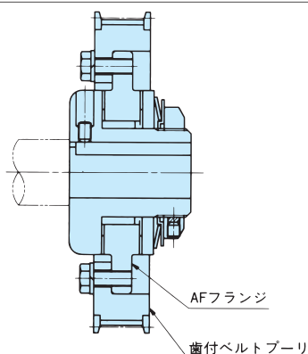
取付例 1
