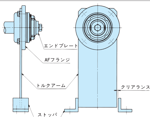
取付例 2
