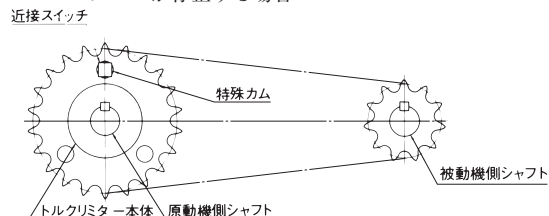
形式 2 被動機械に過負荷がかかって、トルクリミター本体が停止する場合
