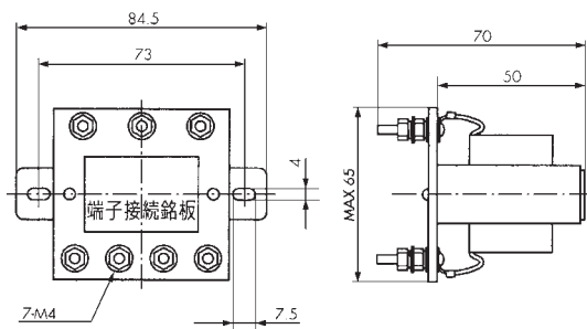
共通形 CT (変流器) TSB COM/TSB COM-A
