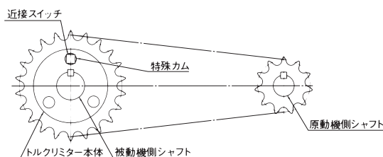
形式 2 被動機械に過負荷がかかって、トルクリミター本体が停止する場合
