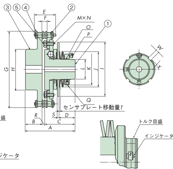
①ショックガード本体 ②TGB スプロケット ③CP スプロケット ④ローラチェーン ⑤六角ボルト
